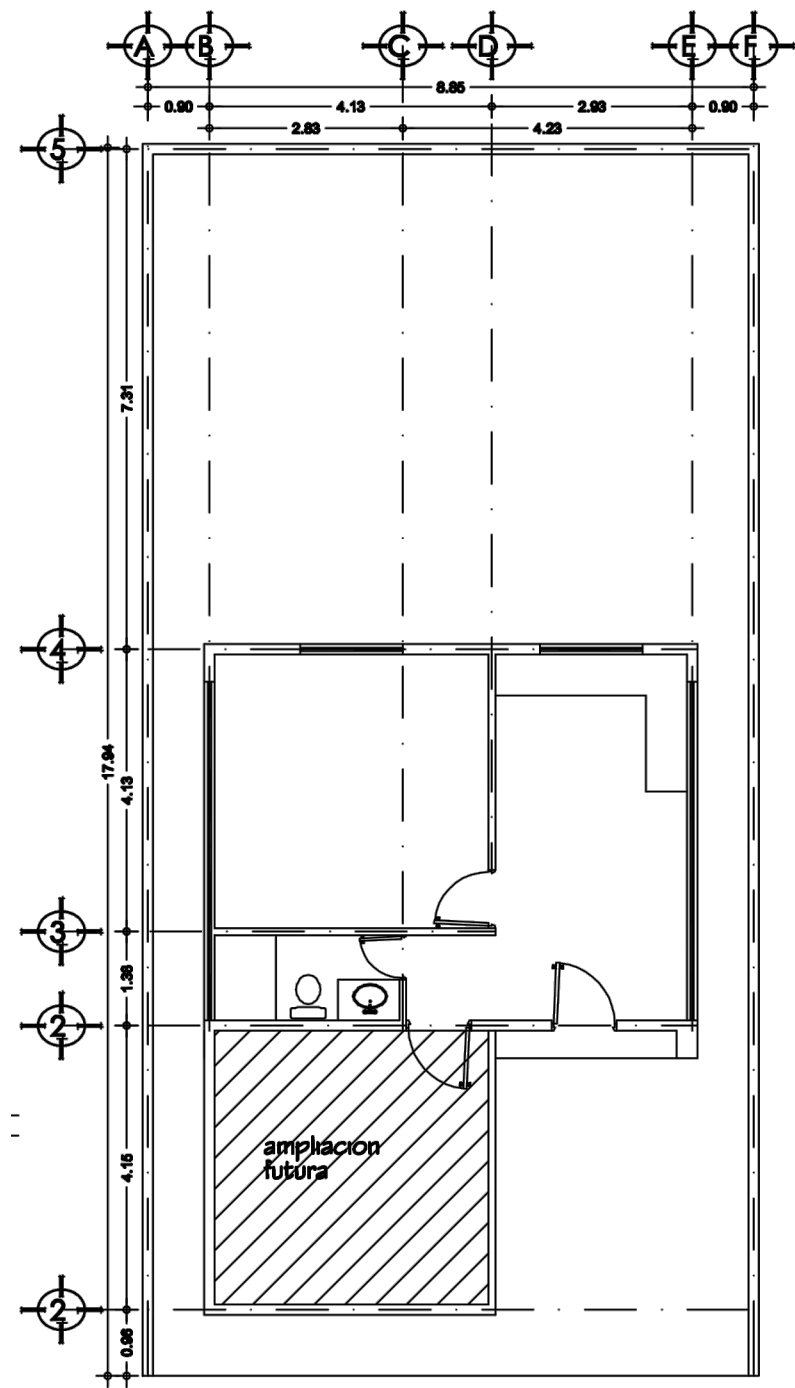
PLANTA
