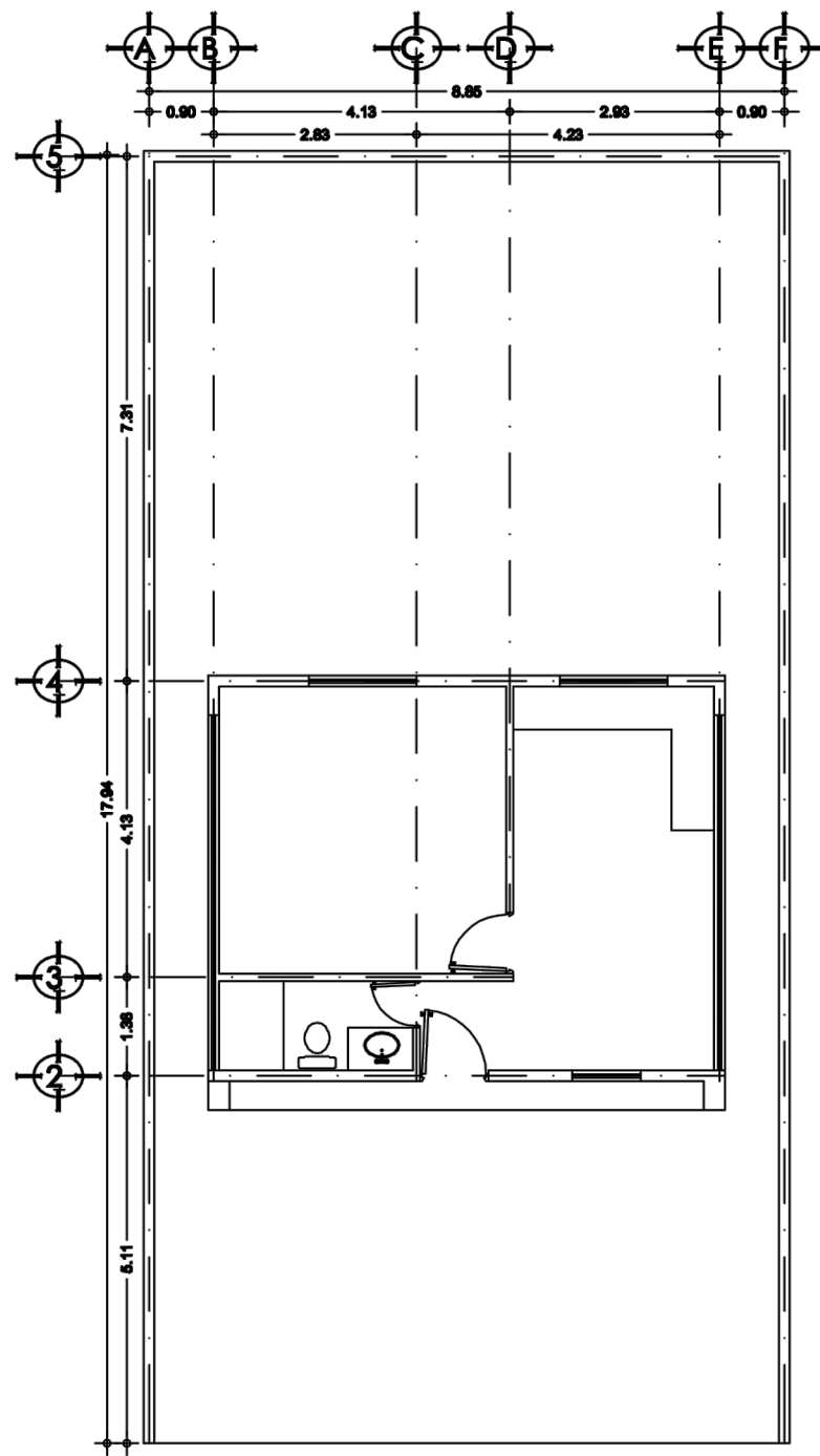
PLANTA
