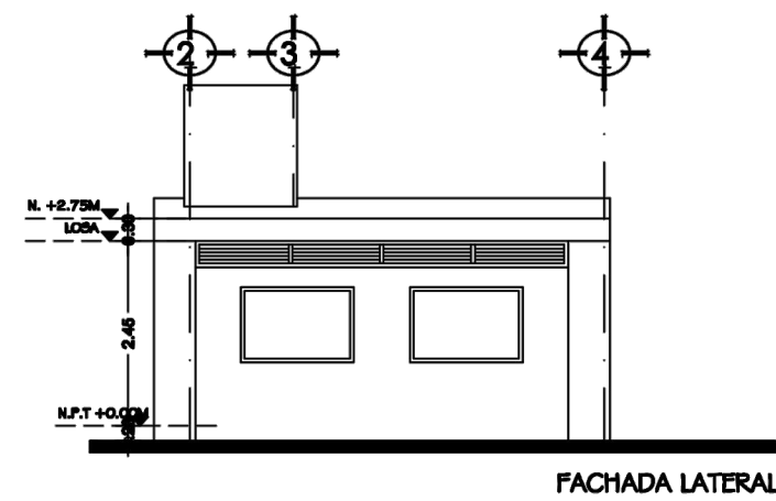
FACHADA LATERAL
