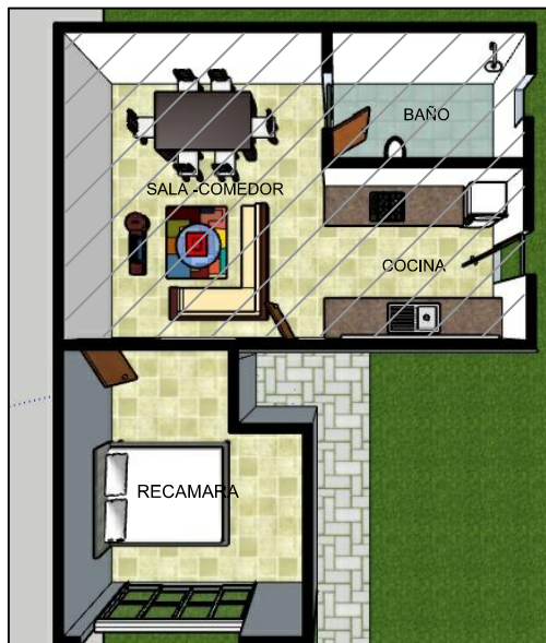
PLANTA ARQUITECTONICA OPCION 1 S/E
